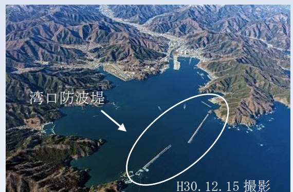
釜石港（完成）
