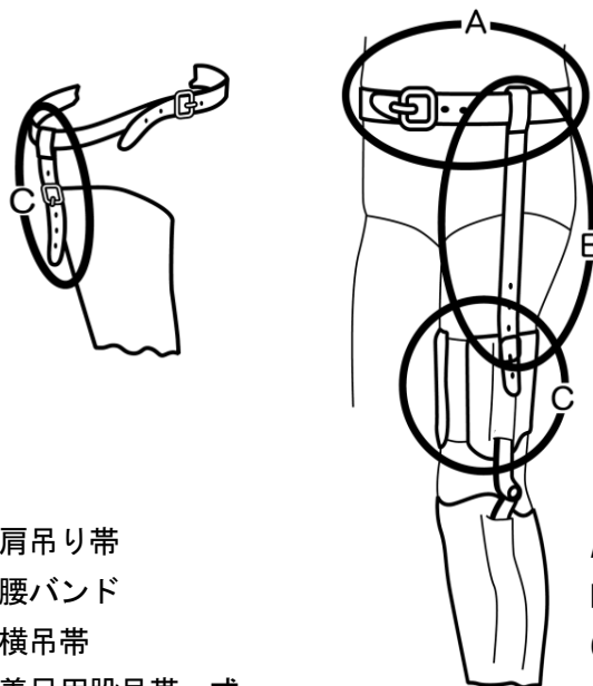
図-22 義足懸垂用部品 （大腿義足・膝義足用）
