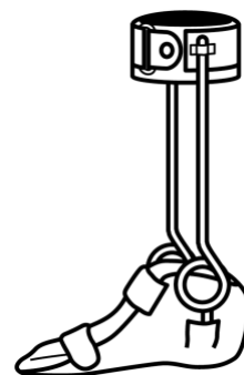
図-40 鋼線支柱 (2単位で算定)
