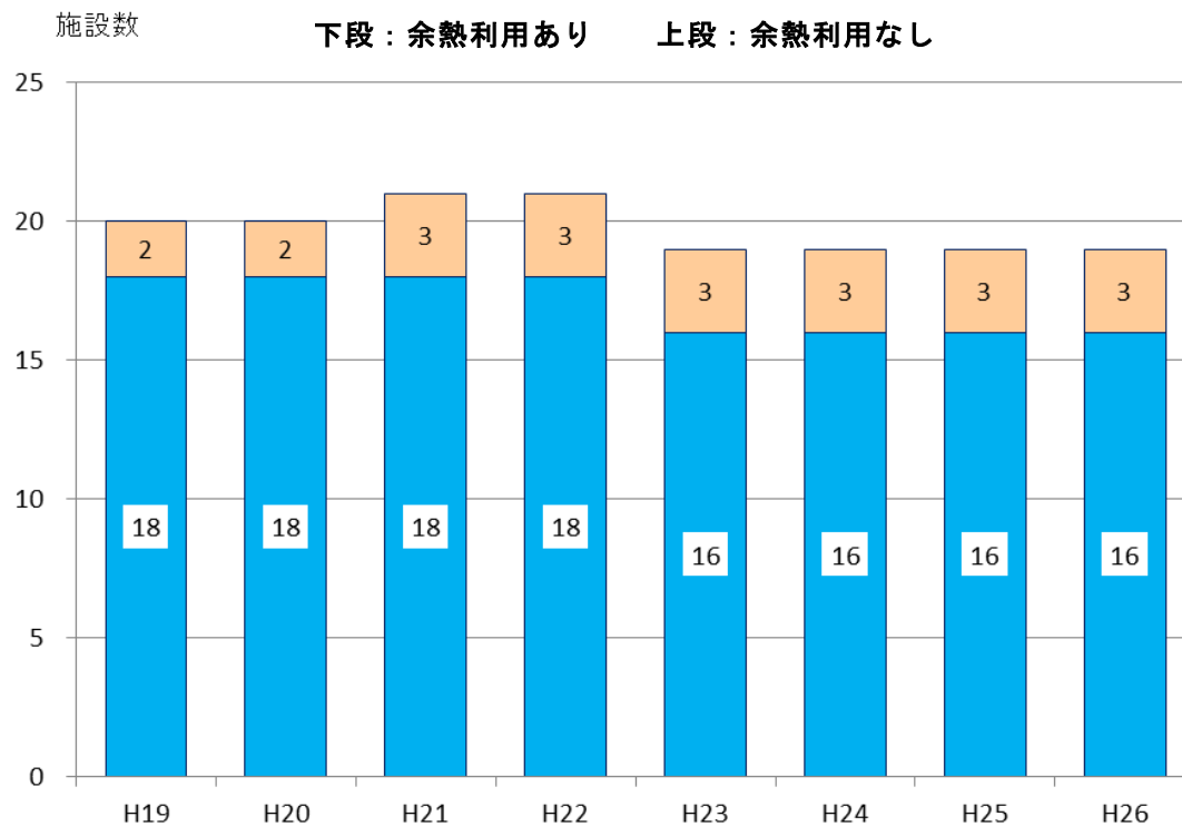
図－１１ ごみ焼却施設の規模別施設数
