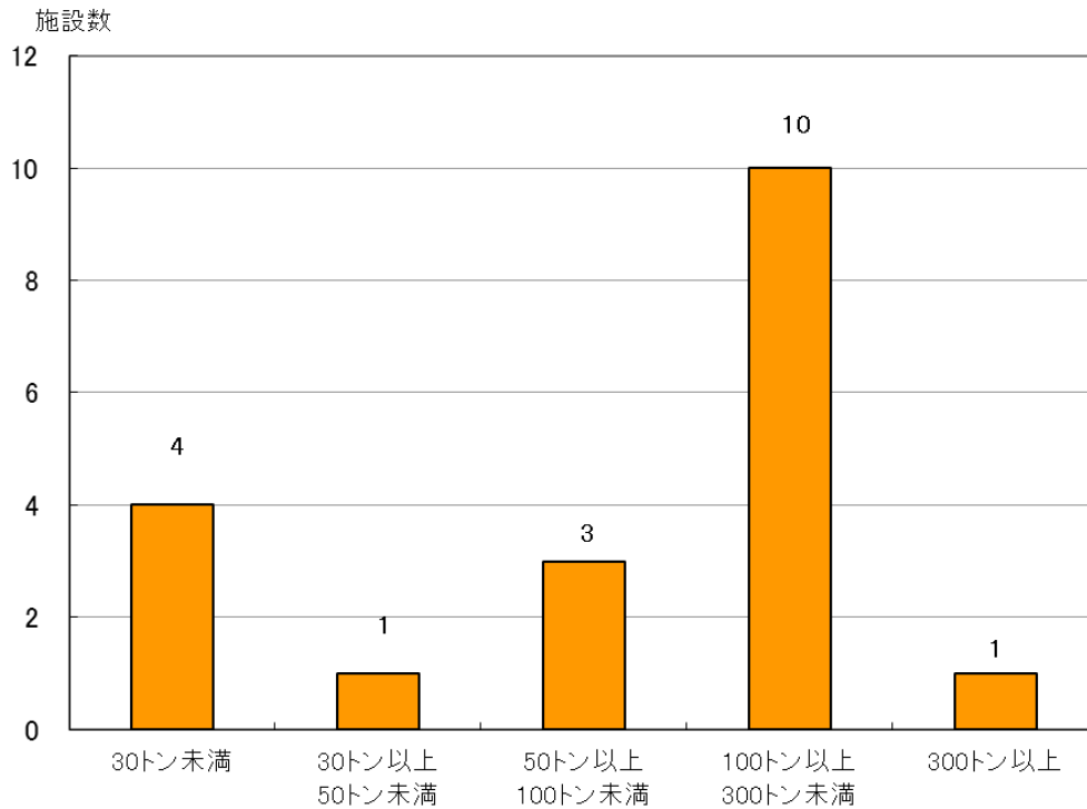
図-10 ごみ焼却施設の規模別施設数
