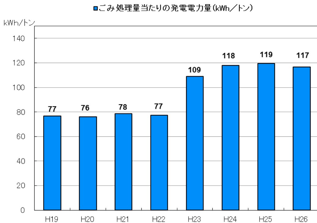
図－12 ごみ処理量当たりの発電電力量
