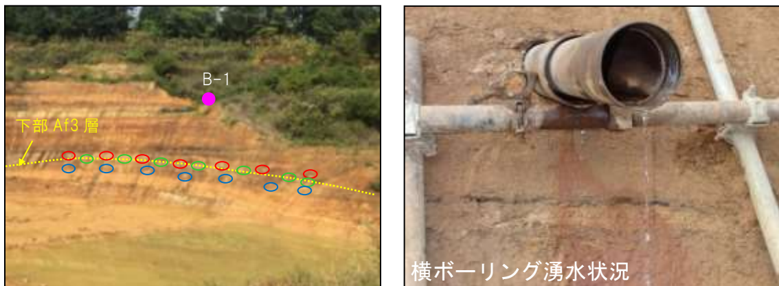
図5 AB地区境界部横ボーリング設置状況
