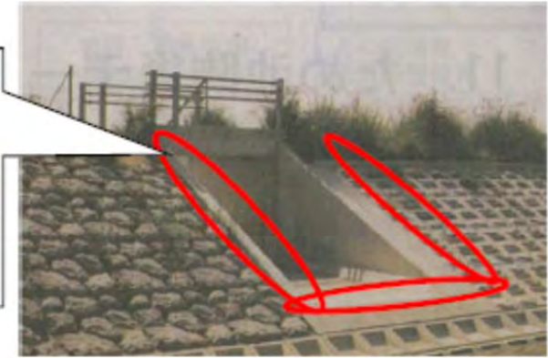
写真11：洪水吐（貯水池側より）
