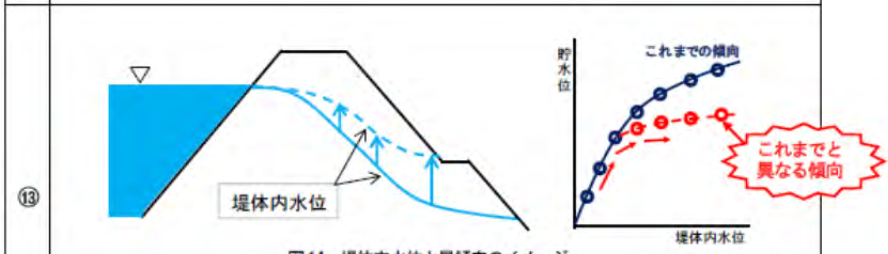
図14：堤体内水位上昇傾向のイメージ
