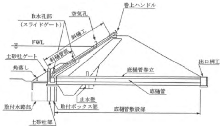
図4：取水施設の構造例
