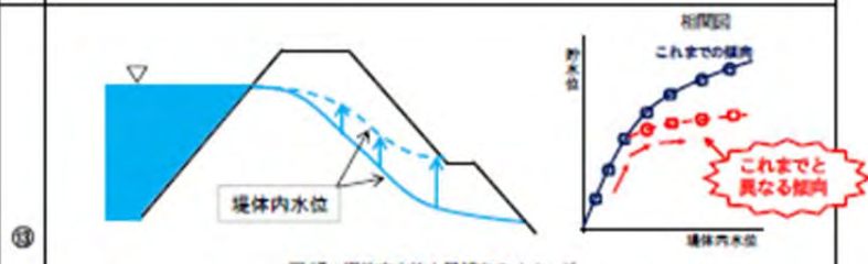
図17：堤体内水位上昇傾向のイメージ
