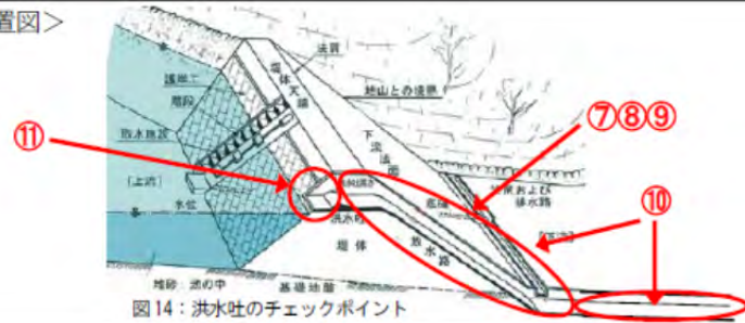
図 14: 洪水吐のチェックポイント
