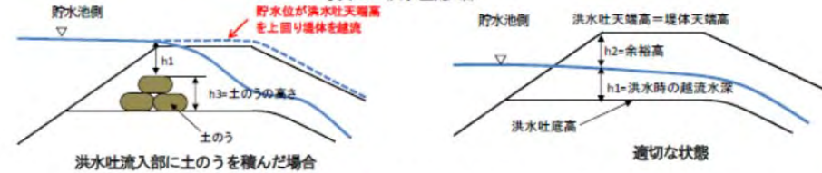
図8：洪水時の水位の違いのイメージ
