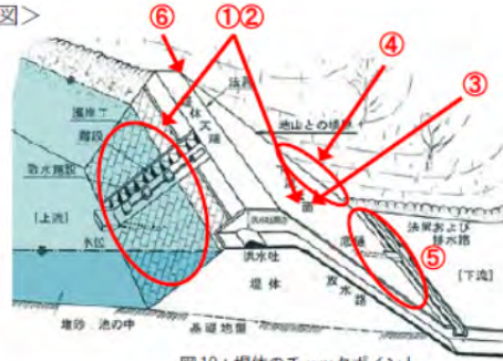
図10：堤体のチェックポイント
