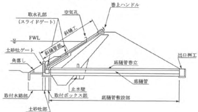
図3：取水施設の構造例
