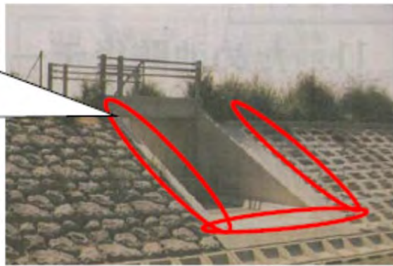
写真10：洪水吐（貯水池側より）
