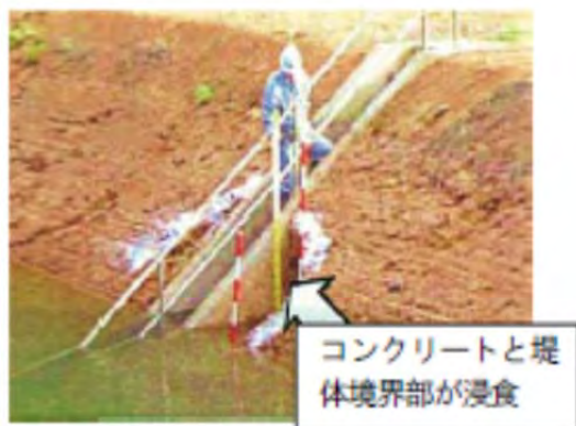
写真12：取水施設
