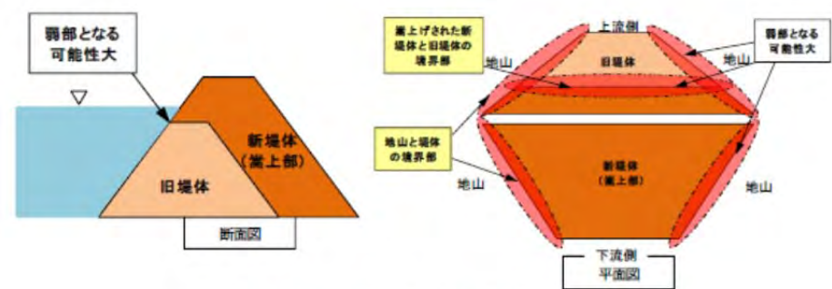
図6：堤体嵩上げした場合の劣化に対する弱部
