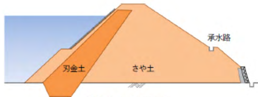
図2 ため池の断面図
