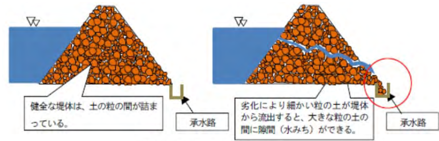
図5：土の細粒分が流出するイメージ
