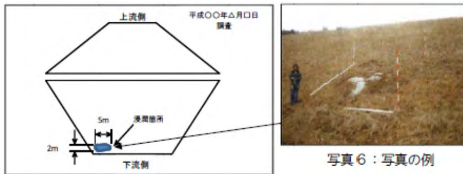
図5：変状箇所のスケッチ
