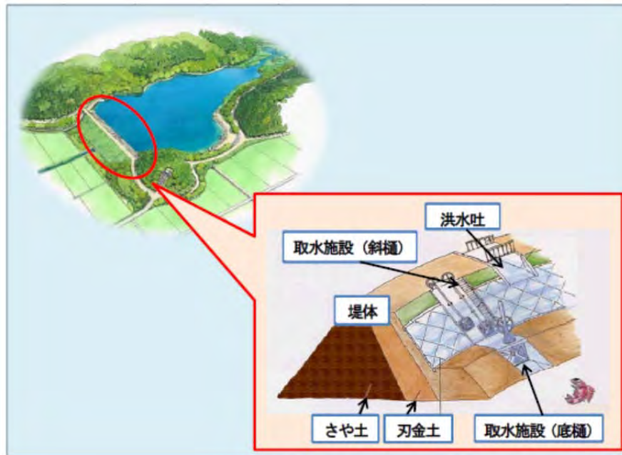
図2：ため池の施設
