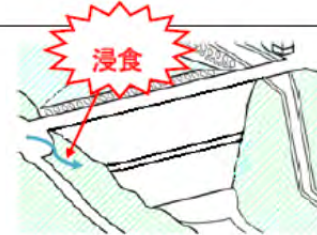
図11:接続道路からの排水による堤体の浸食
