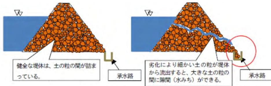
図6：土の細粒分が流出するイメージ
