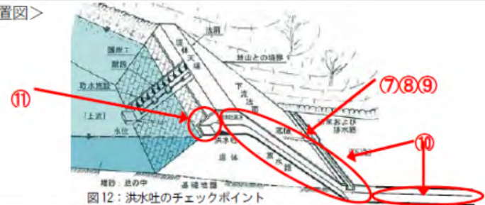
図 12: 洪水吐のチェックポイント
