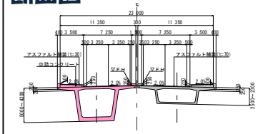
断面図 (下り線)
