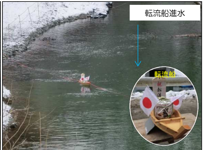
転流のようす (上流側)
