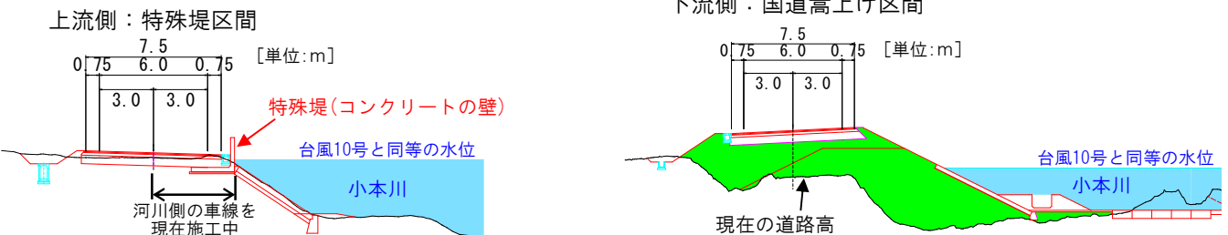
特殊堤区間の工事状況
