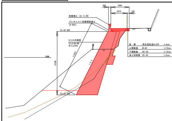
標準横断面
