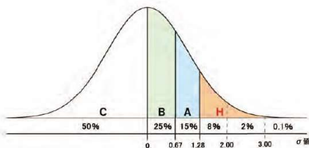
図2 母集団の分布モデル
