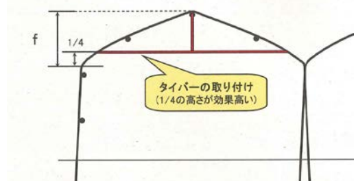
タイバーによる肩部の補強事例
