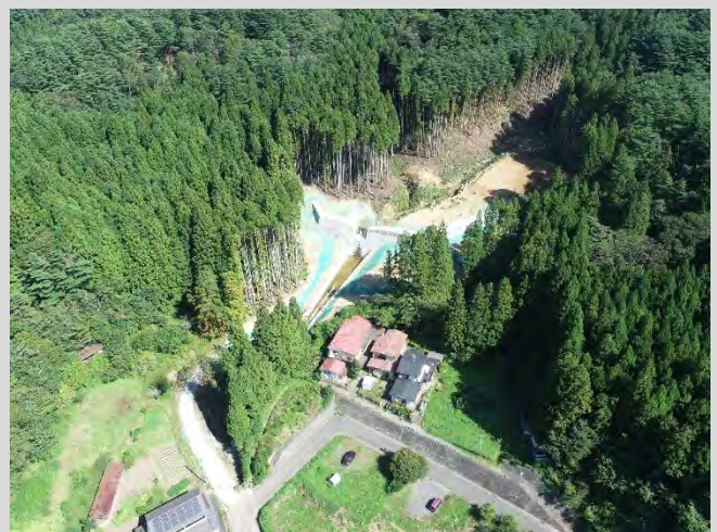
砂防堰堤完成状況(令和4年11月完成)
