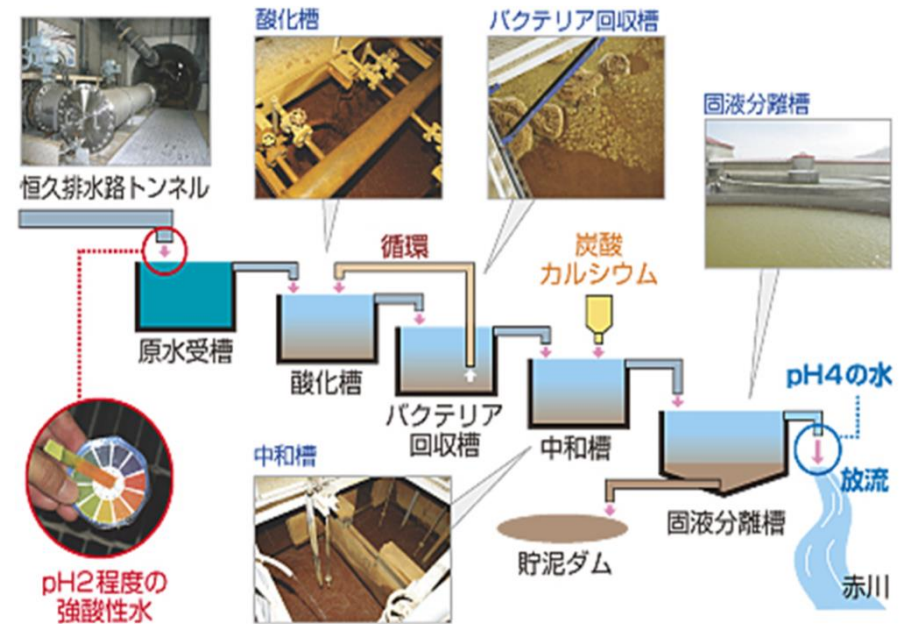
強酸性で重金属を多量に含む坑廃水を微生物（バクテリア）の力を利用して効率的に中和処理している仕組みを分かりやすくお伝えします。
