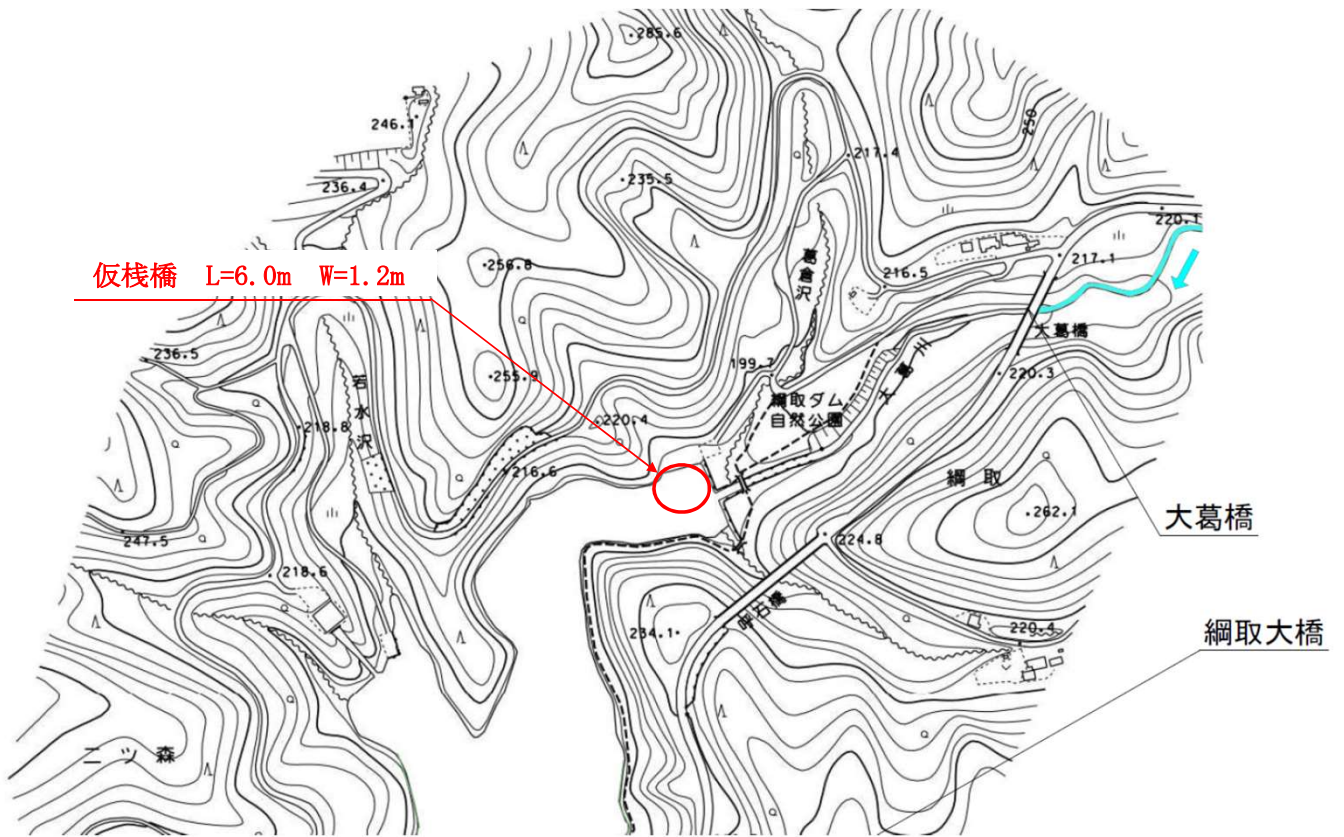
仮棧橋 位置図(参考図)
