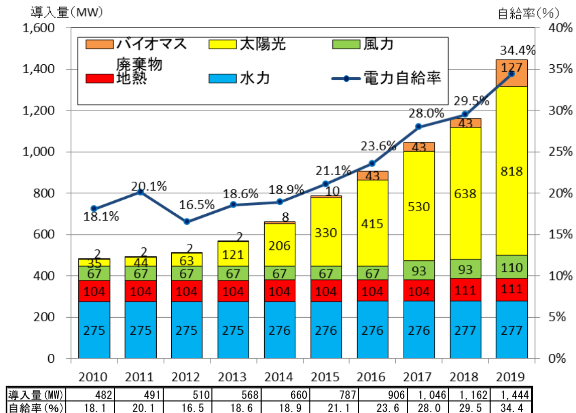
図 4-13 再生可能エネルギー（電気）の導入状況
