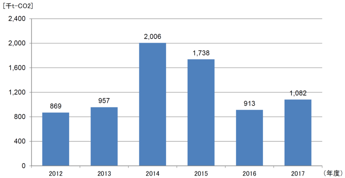
図 4-17 森林吸収量の推移
