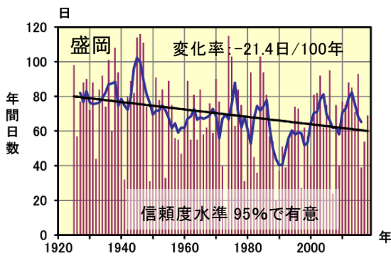
図7-4 盛岡日最深積雪5cm以上の年間日数（寒候年 1 ）の推移 棒グラフは各年の日最深積雪5cm以上の年間日数、折線は5年移動平均値、直線は長期変化傾向を表す。
