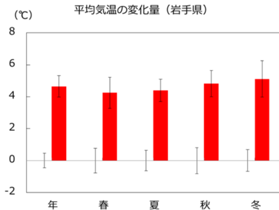
図7-6 岩手県の年平均気温の変化量 現在気候（1980～1999年の20年平均値）に対する将来気候（2076～2095年の20年平均値）の変化量（°C）。気象庁によるIPCCのRCP8.5シナリオに基づくシミュレーション結果（気象庁，2017）を基に作成。
