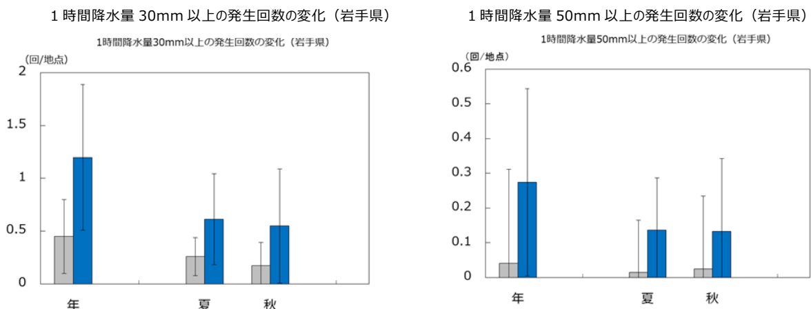
図 7-8 1 時間降水量 30 mm 以上(左)および 50mm 以上(右)の 1 地点あたりの年間発生回数の変化
