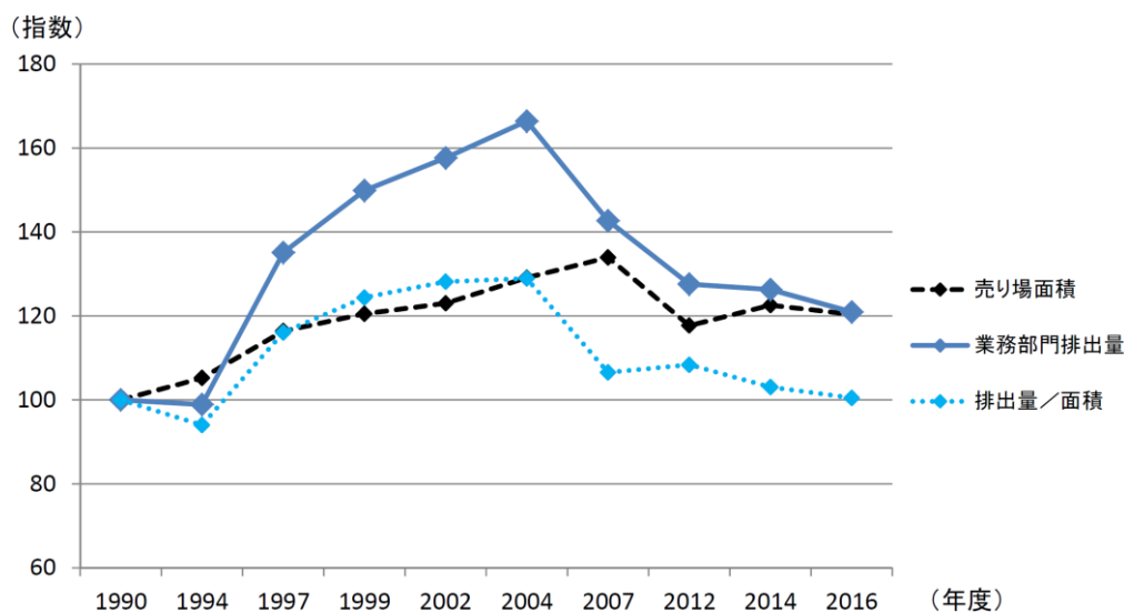
図 4-11 売り場面積当たりの二酸化炭素排出量の推移
