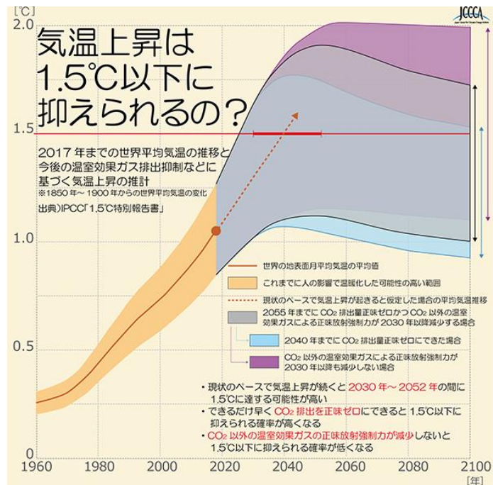
図3-4 IPCC「1.5℃特別報告書」
