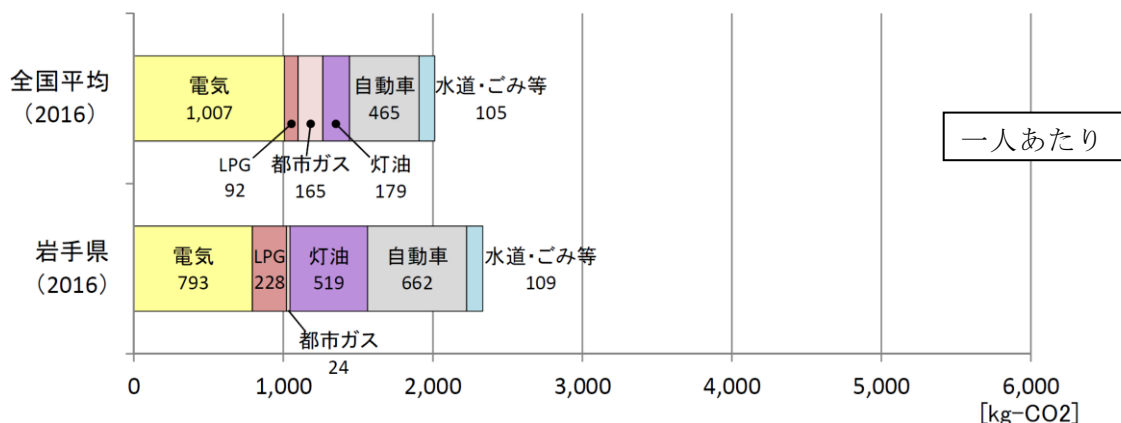
図 4-7-2 世帯の一人当たりの二酸化炭素排出量の状況
