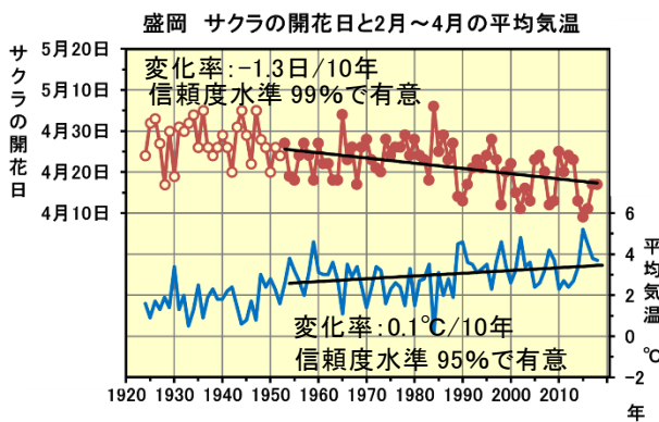
図7-5 盛岡のサクラ開花日と2月～4月の3か月平均気温の推移
