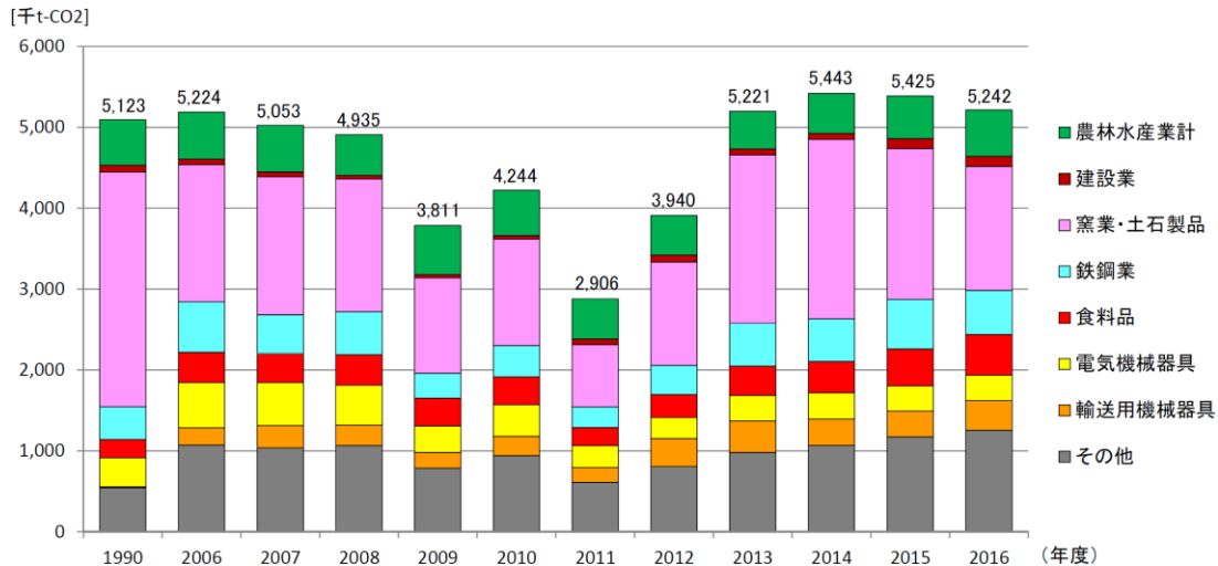
図4-8 業種別二酸化炭素排出量の推移
