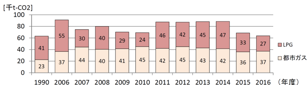
図 4-10-2 民生業務部門のエネルギー種別二酸化炭素排出量の推移 (ガス内訳)
