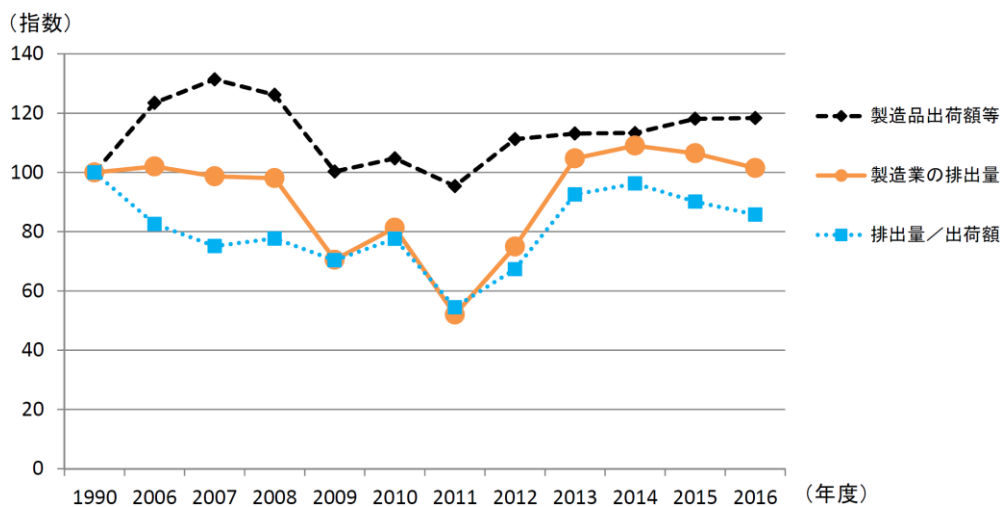
図4-9 製造業品出荷額当たりの二酸化炭素排出量
