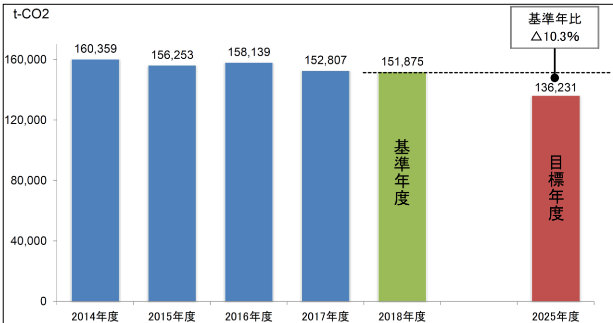
図 6-1 温室効果ガス排出量と削減目標値
