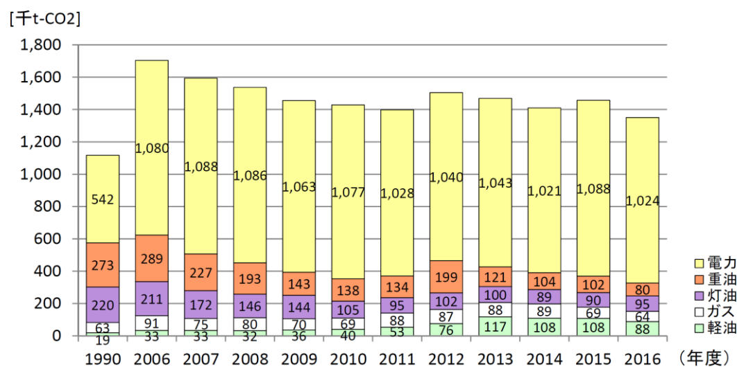
図 4-10 民生業務部門のエネルギー種別二酸化炭素排出量の推移
