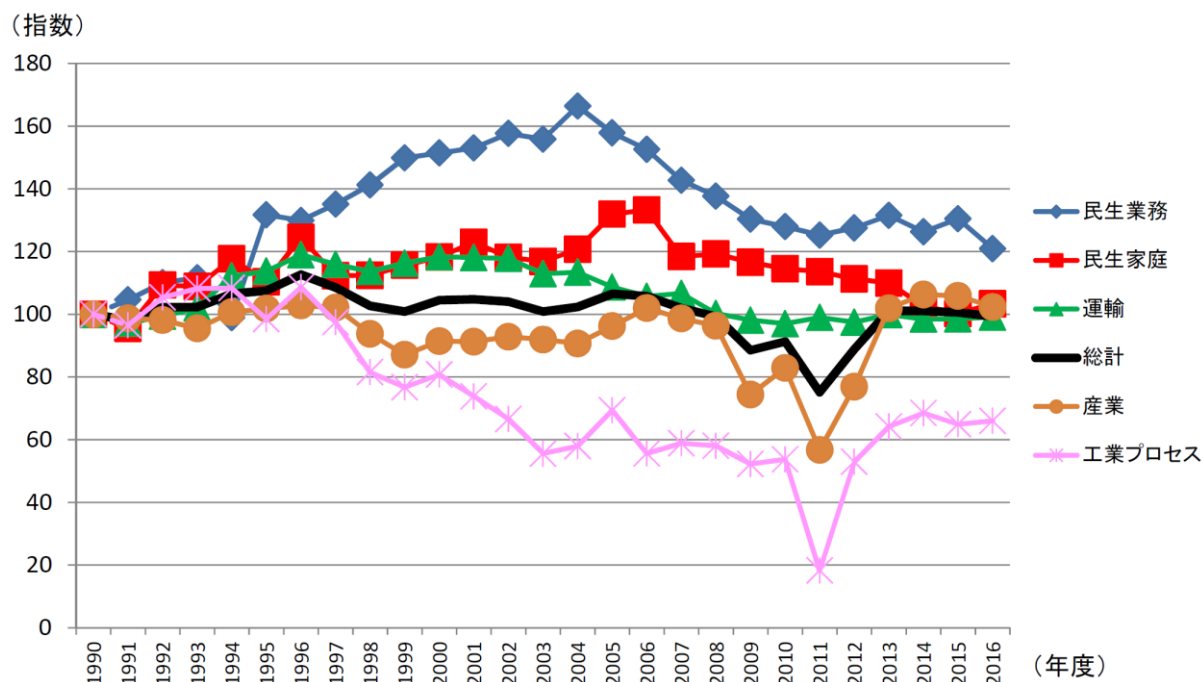
図 4-3 二酸化炭素排出量における部門別の基準年比の推移
