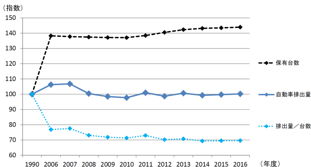
図 4-13 自動車保有台数当たりの自動車二酸化炭素排出量等の推移
