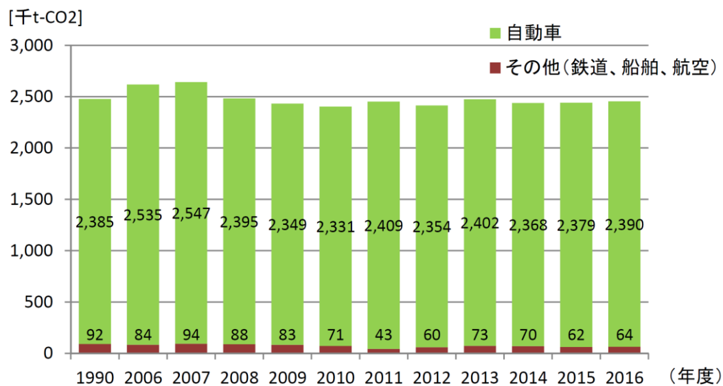
図 4-12 輸送種別二酸化炭素排出量の推移
