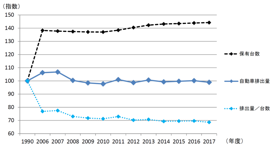
図 4-14 自動車保有台数当たりの自動車二酸化炭素排出量等の推移
