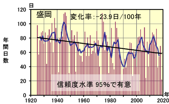
図7-4 盛岡日最深積雪5cm以上の年間日数（寒候年 1 ）の推移
