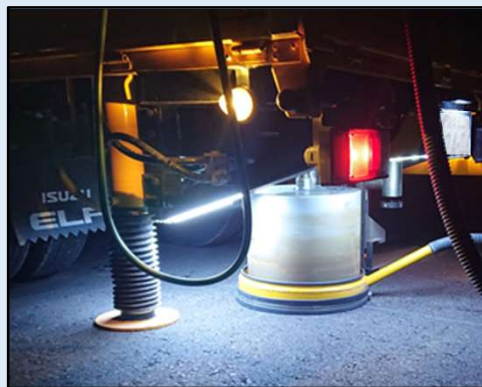
① コアカッターによる削孔(1) (事前にテストボーリング実施)
