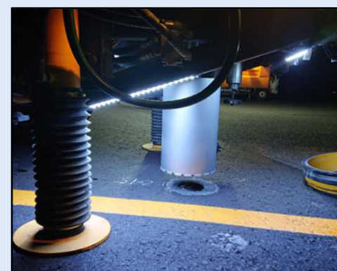
③ コアカッターによる削孔
