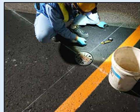
⑥ 灯器設置完了 （この後、樹脂注入作業）
