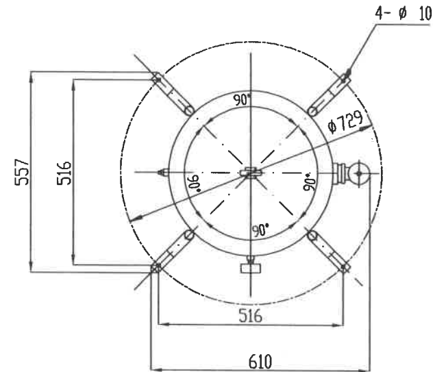
矢視 A
