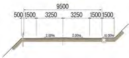
標準断面
