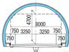
トンネル断面
