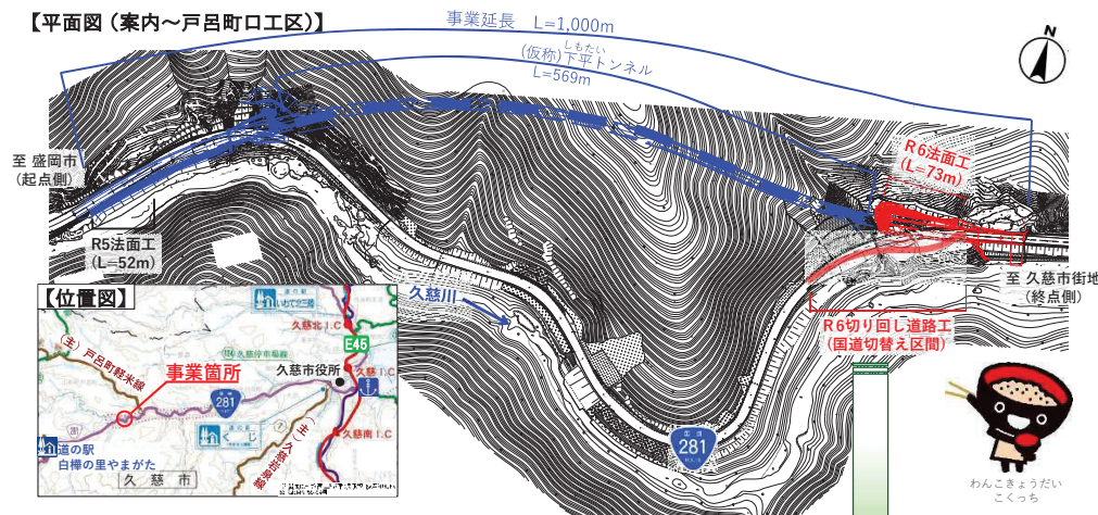
【平面図（案内～戸呂町口工区）】
