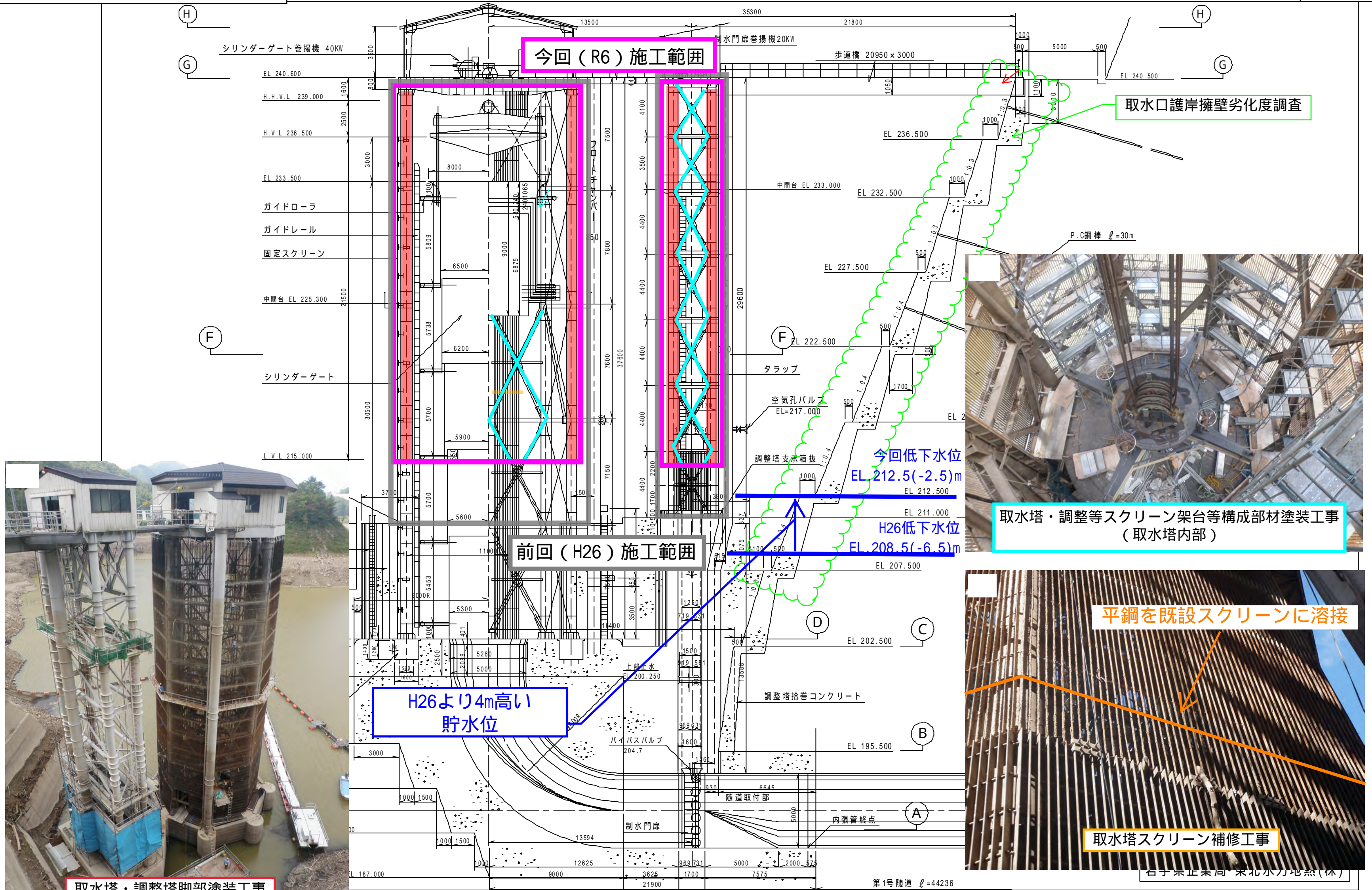
取水塔・調整塔脚部塗装工事
