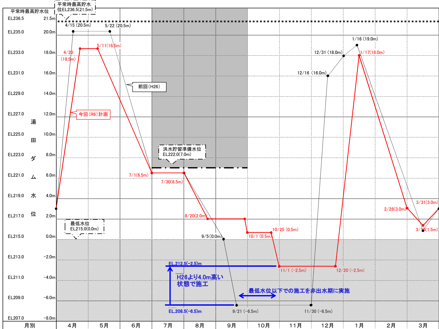
令和6年度 湯田ダム水位運用計画表（前回（H26）定期点検及び修繕工事の時との比較）
