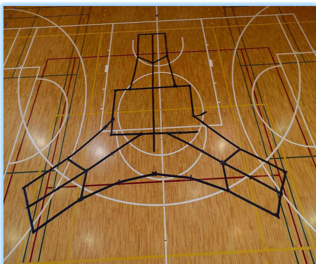
トータルステーションを用いて、参加生徒全員で校章を体育館に描画
