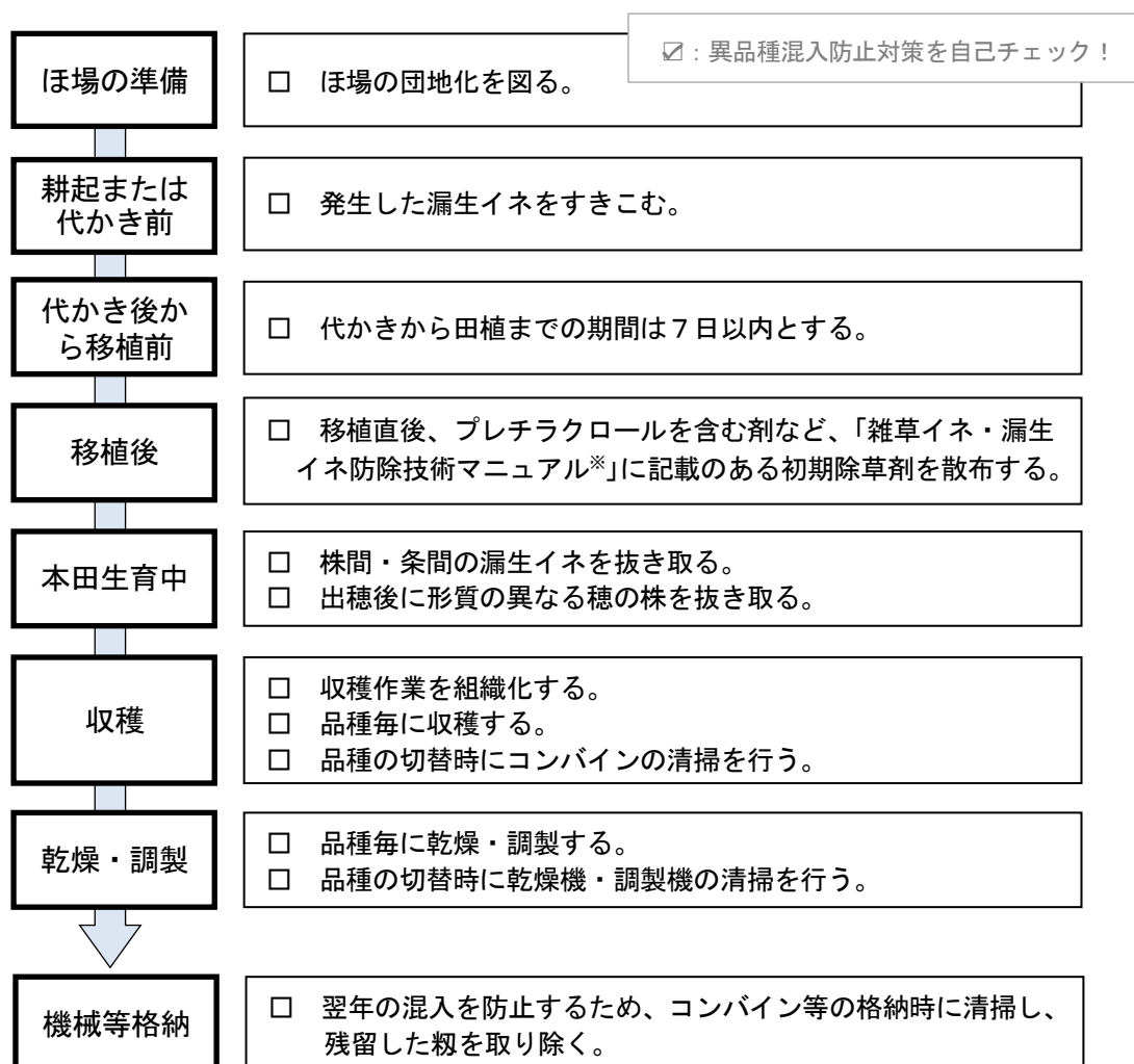
図12 異品種混入防止対策の作業フロー
