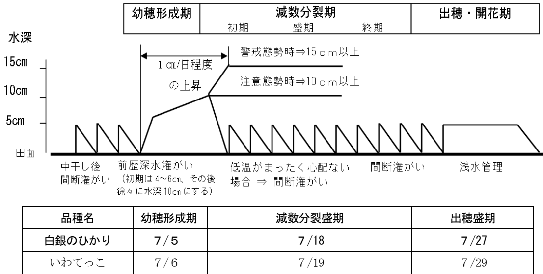
図9 中干し後の水管理の模式図
