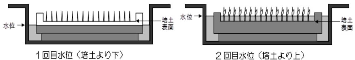
図4 プール育苗の水管理
