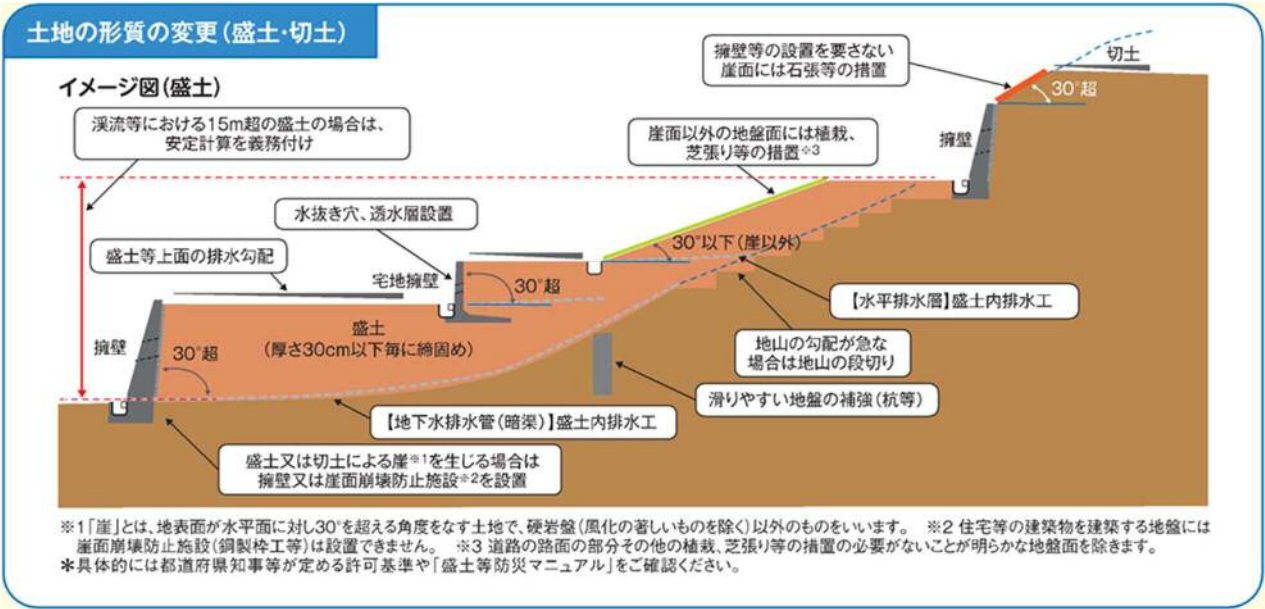
図ー13 盛土及び切土の各種施設の概念図
