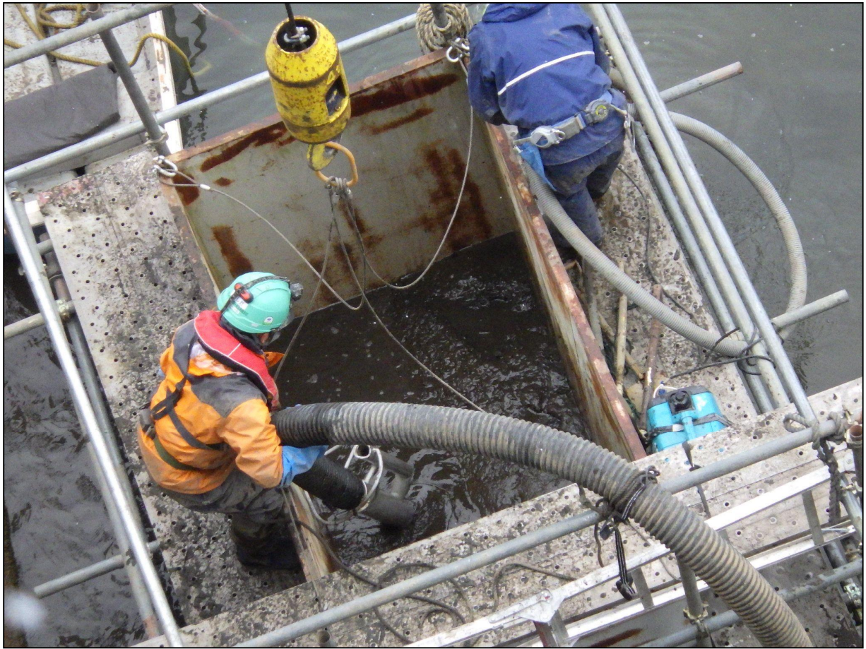
作業状況 5 土砂（泥水）吸引
