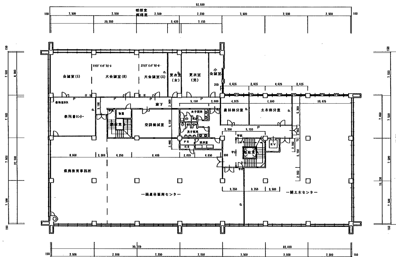
3階 平面図 1/200
