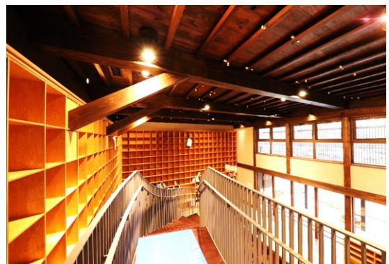
既存大梁は新材と継いで再利用している
