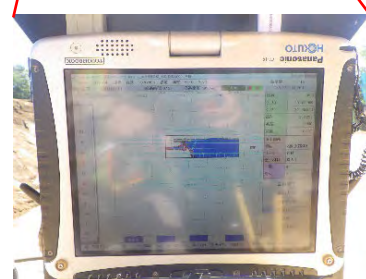
I C T 建設機械による施工状況
