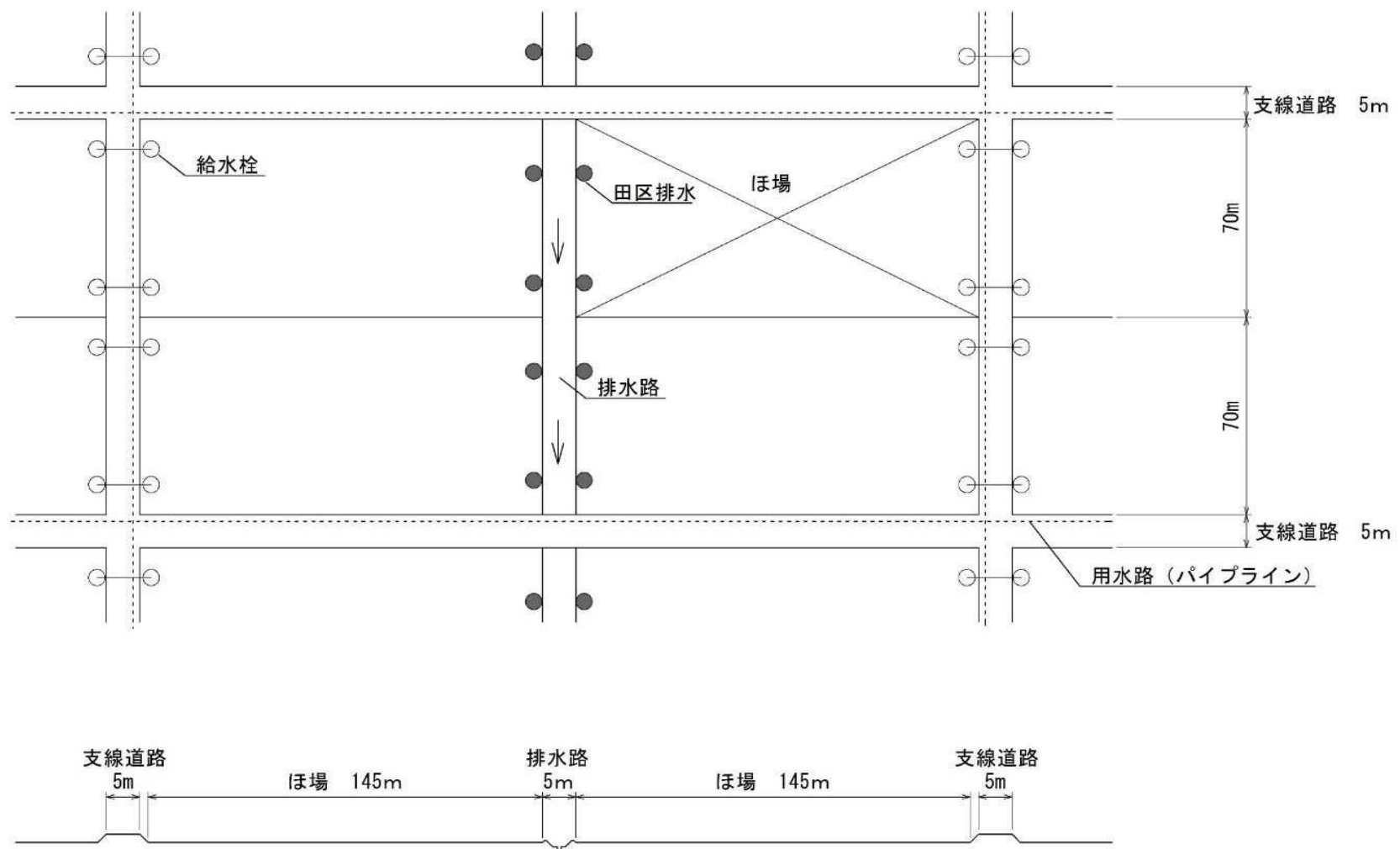
末端道水路配置図
