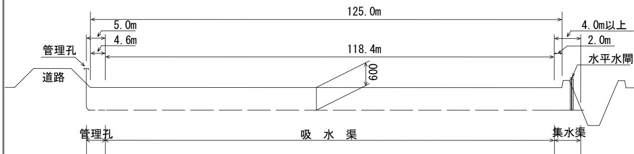
縦断図
