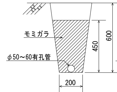
管理孔断面図
