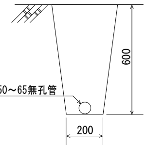
集水渠断面図
