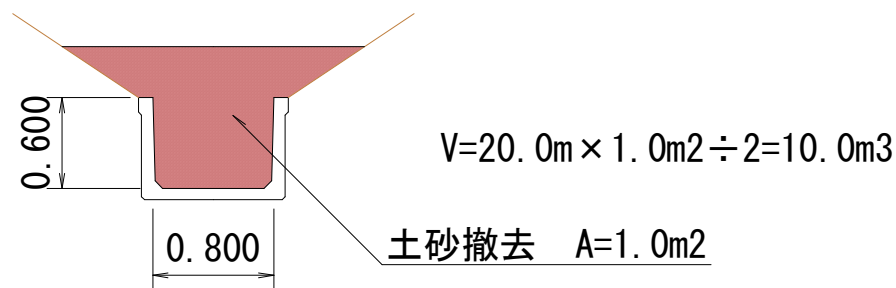
標準図 (S=1 : 50)
