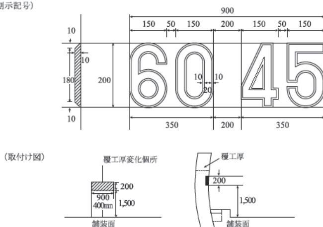
図10-6-1 覆工厚変化箇所の刻示標準図
