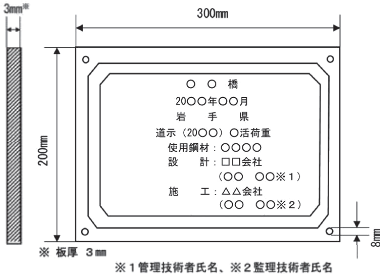
図3-2-2 銘板の寸法及び記載事項
