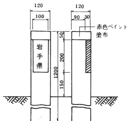
图 用地境界杭
