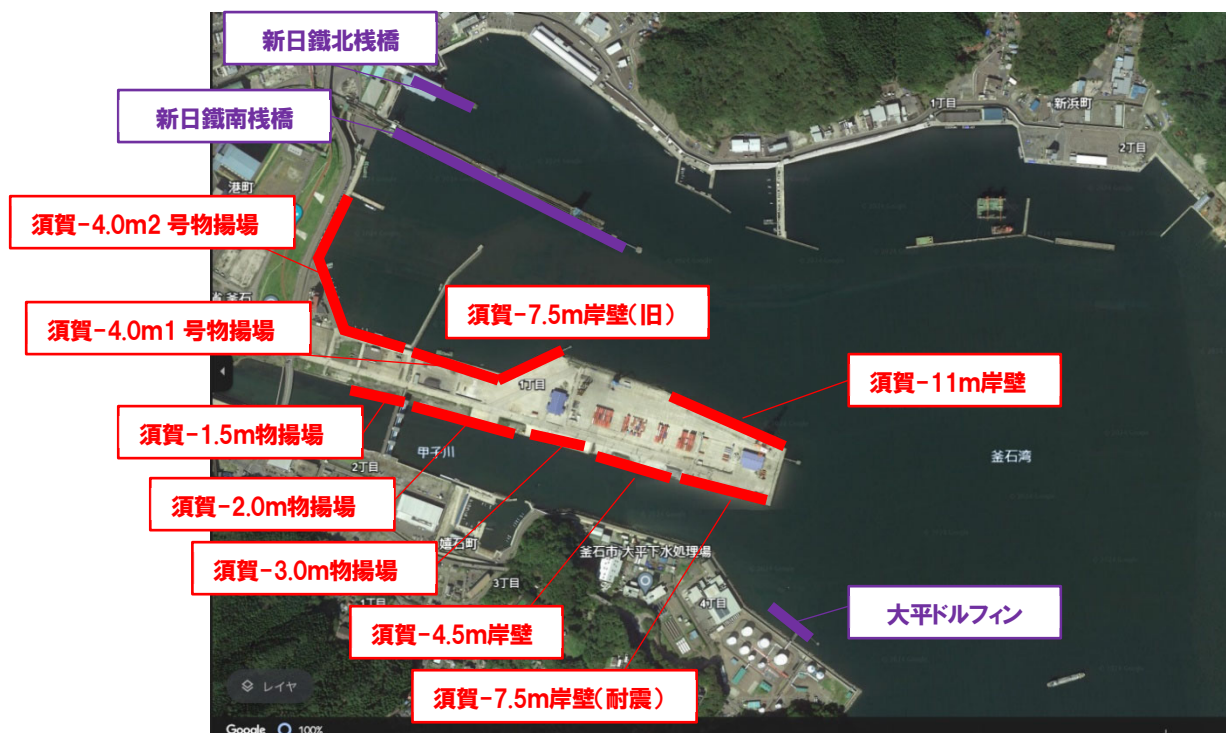
図 1-3 係留施設位置図
