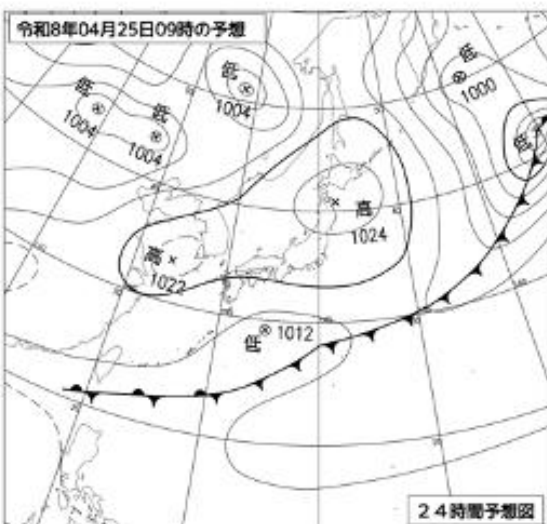
4月25日 09時 の予想天気図
